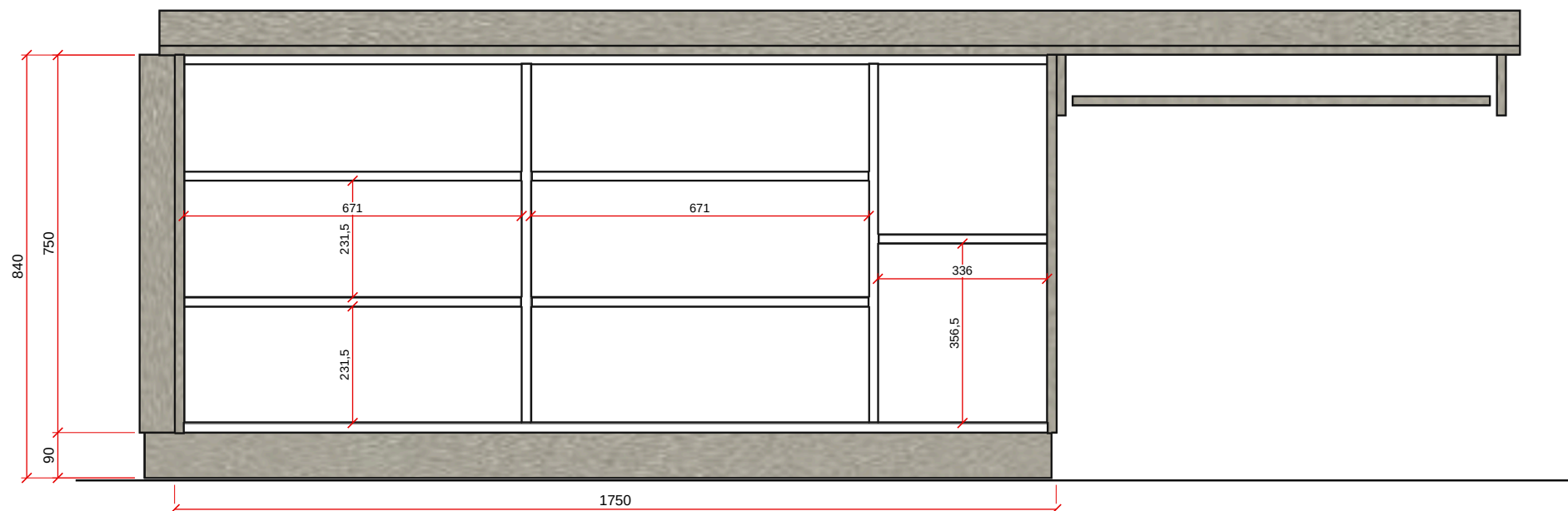
VISTA A - ESC. 1:12.5
